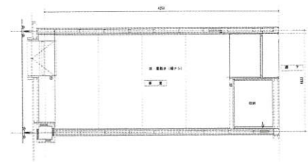
客室平面詳細図 S=1/100
